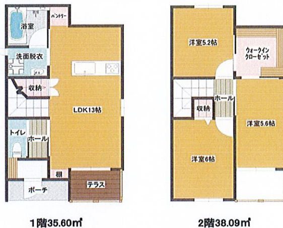
リコメリアB,C,D棟 延床面積73.69㎡
